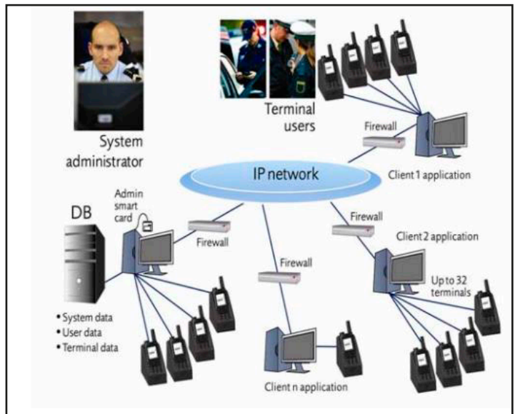
Server/klient konfiguration
