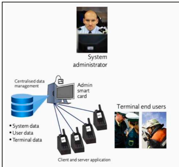
Lokal konfiguration
